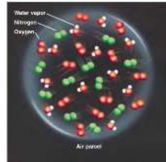
Fig. 1: Moist air parcel
